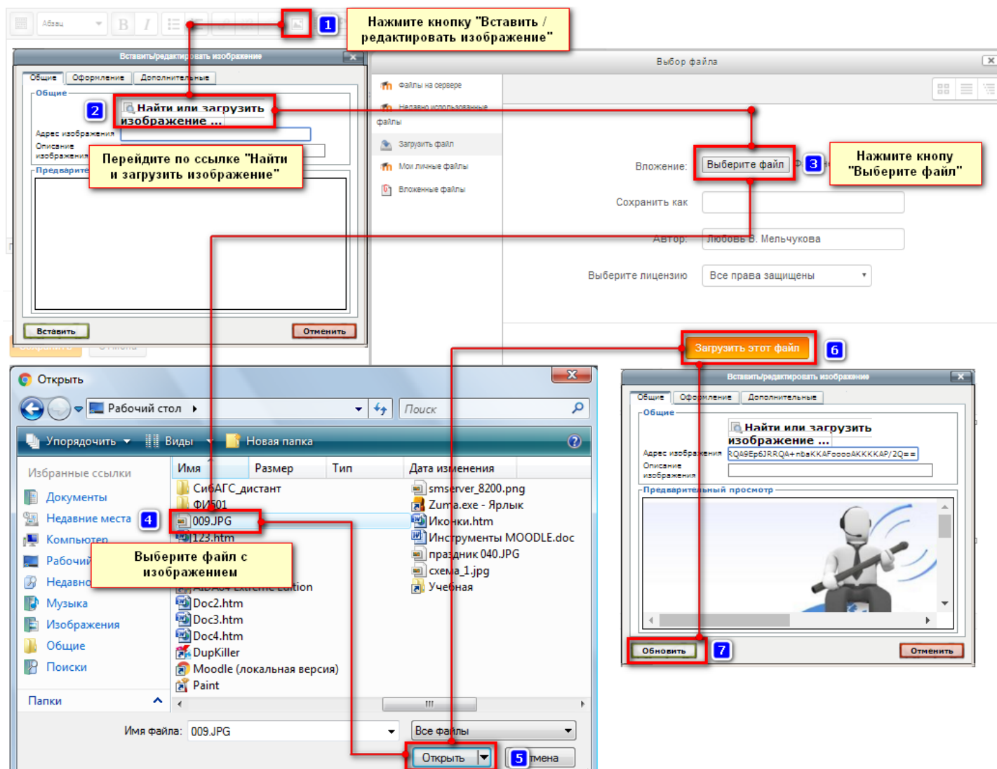
Рис.3. Загрузка изображения
